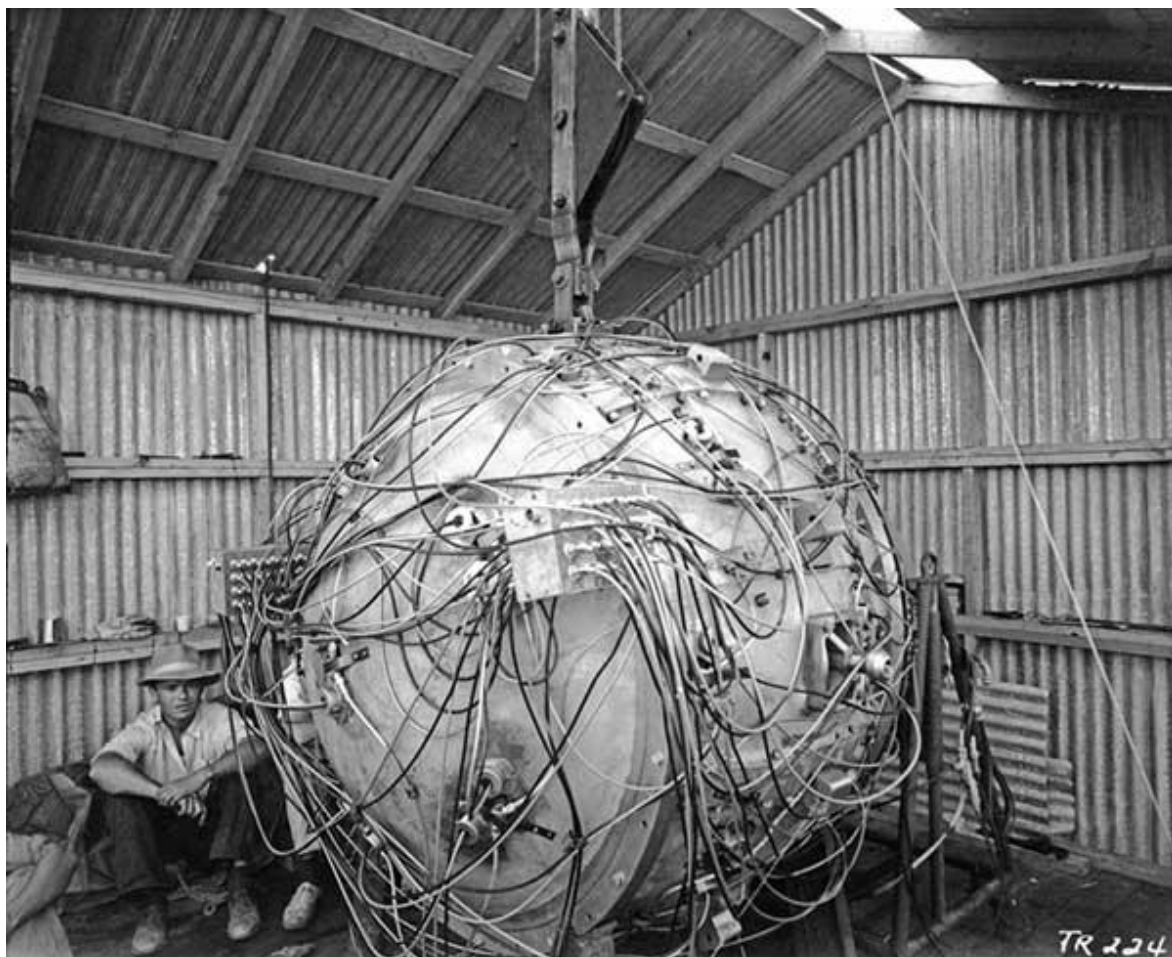
Zařízení s kódovým označením Trinity (Svatá trojice), se kterým byl proveden první jaderný test 16. července 1945 v Novém Mexiku
